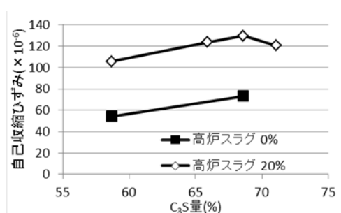
図-3 C 3 S 量と自己収縮の関係
