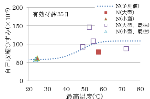
図-2 最高温度と自己収縮の関係
