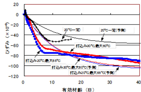
図-1 自己収縮ひずみの経時変化
