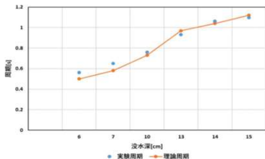
図 7 形状Aの固有振動周期と水柱の水位の関係
