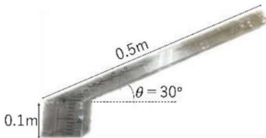
図 5 水位の影響評価に利用した実験模型
