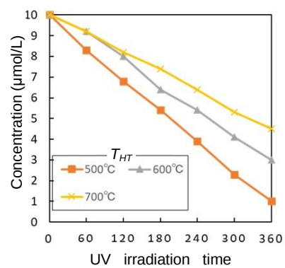
図6 \text{TiO}_2 薄膜（加熱・急冷処理後）のメチレンブルー脱色試験結果 ( T_{HT} : 加熱処理温度)
