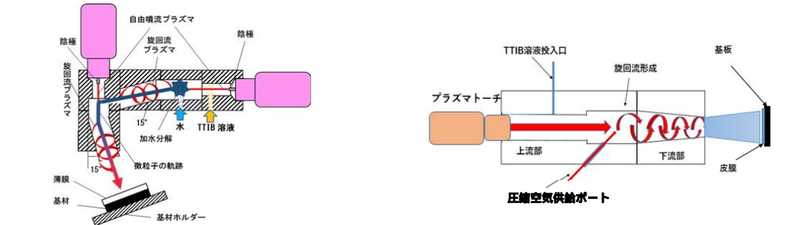
a) クロスフロー型複合プラズマトーチの模式図 b) 旋回空気流導入型シングルトーチの模式図
