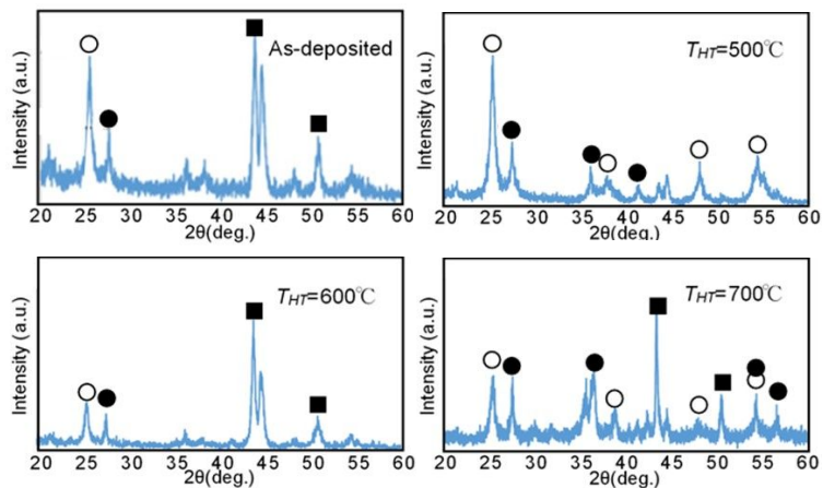
図5 As-deposit 及び加熱・急冷処理後の \text{TiO}_2 薄膜の X 線回折結果
